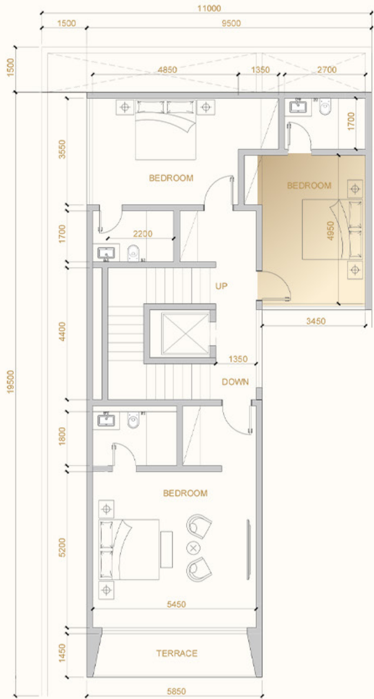
Bedroom 2
